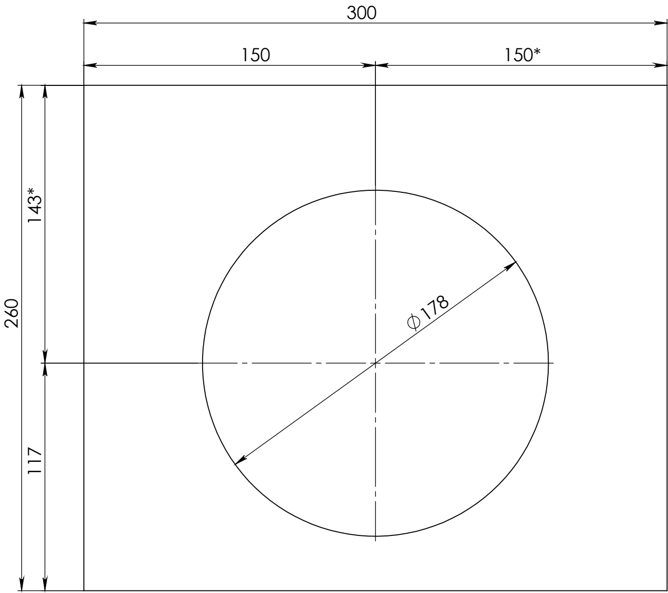
Экран динамика
