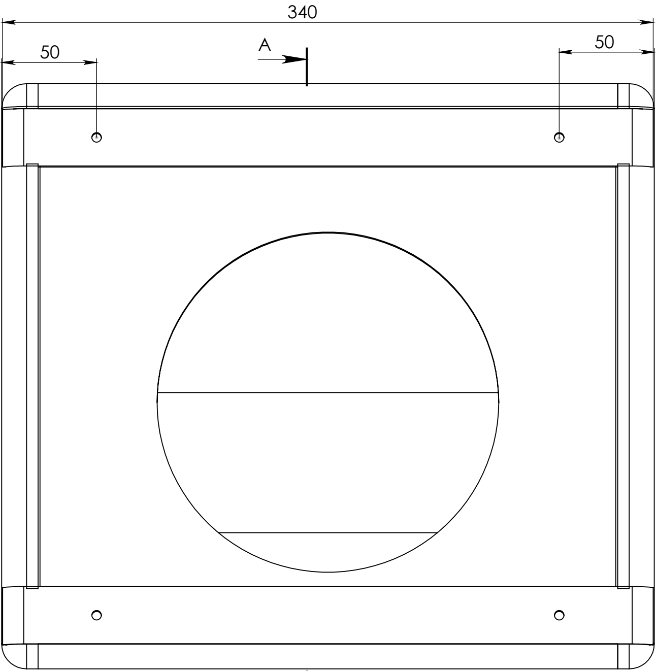
Вид спереди
